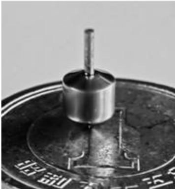
「マイクロコマ」直径4mm0.4g 小さいのに1分半も回転するよ
